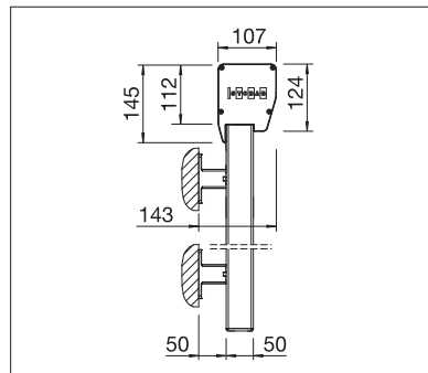
Wandmontage mit eckigem Kasten und Führungsprofil
