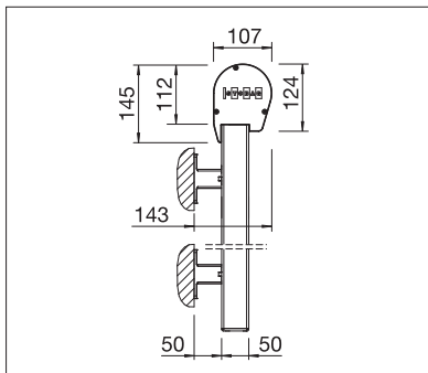
Wandmontage mit rundem Kasten und Führungsprofil
